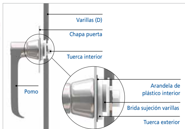
Tirador con cerradura (K1) (puerta derecha)
